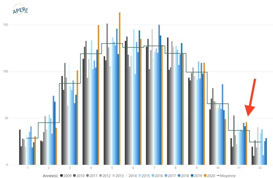
Productivité mensuelle photovoltaïque [kWh/kWc]
